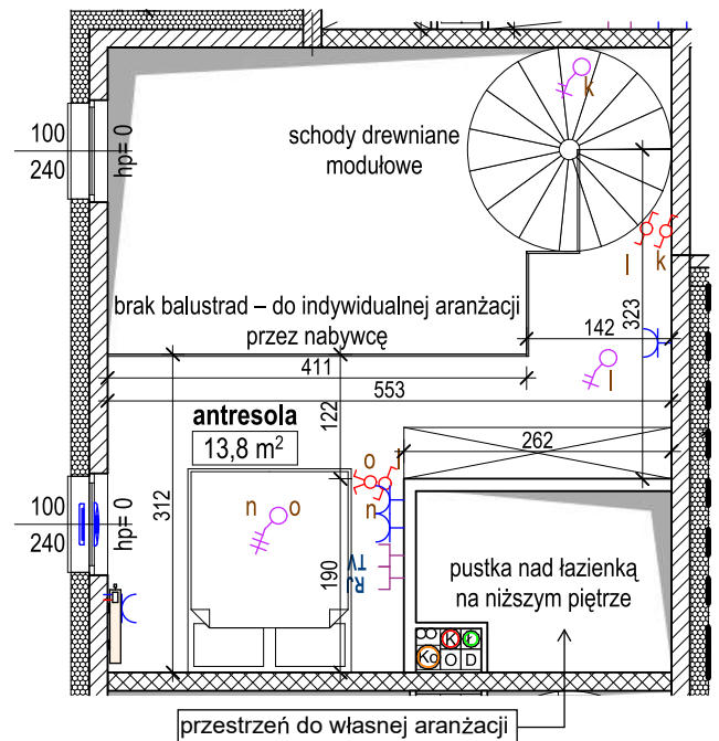
RZUT ANTRESOLI
