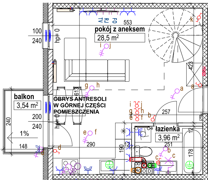
RZUT 3 PIĘTRA
