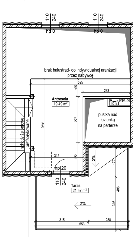
RZUT ANTRESOLI MIESZKANIA
